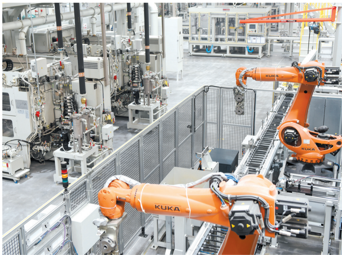
北汽集团零部件轻量化基地引进具有国际先进水平的生产设备及仪器,致力建设一个现代化、数字化、自动化、智能化的先进工厂。
