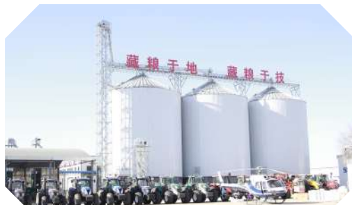
邹平供销社为农服务综合体智能化粮食立筒仓储粮达9000吨。
